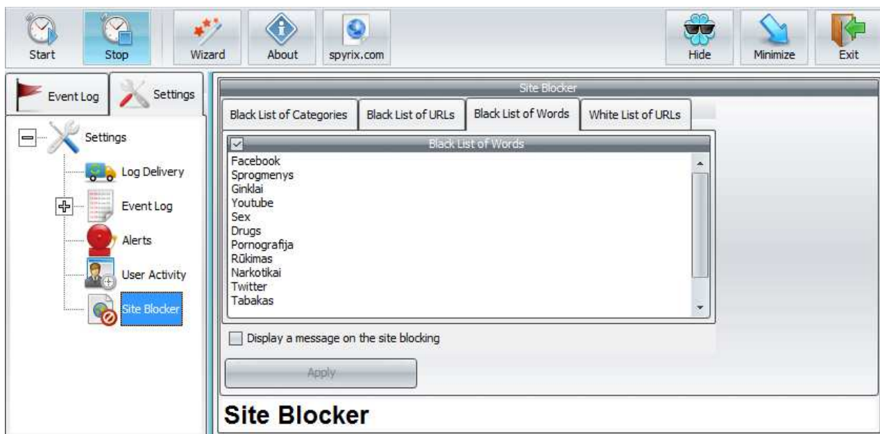
5 pav. Interneto turinio filtravimas pagal raktinius žodžius
